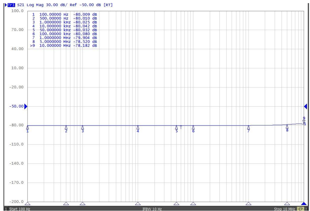
CCM 0210M卡式宽带电流监测钳s21曲线
